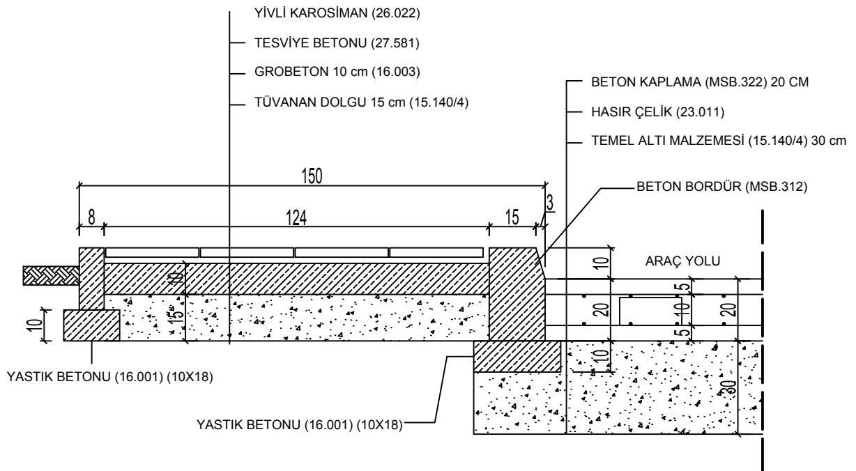
B DETAYI (YAYA YOLU - BETON ARAÇ YOLU KESİTİ) ÖLÇEK : 1/10
